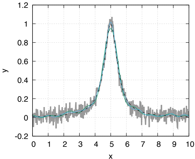
Noisy breit wigner signal
